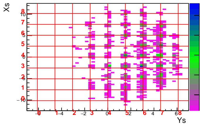
Run 3593 Foil 13.3 DelCut -6.0
