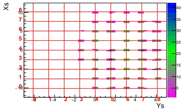
MC Run 3610 Foil 13.3 DelCut -9.0
