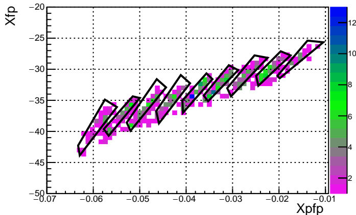
Run 3610 Foil 13.3 DelCut -9.0
