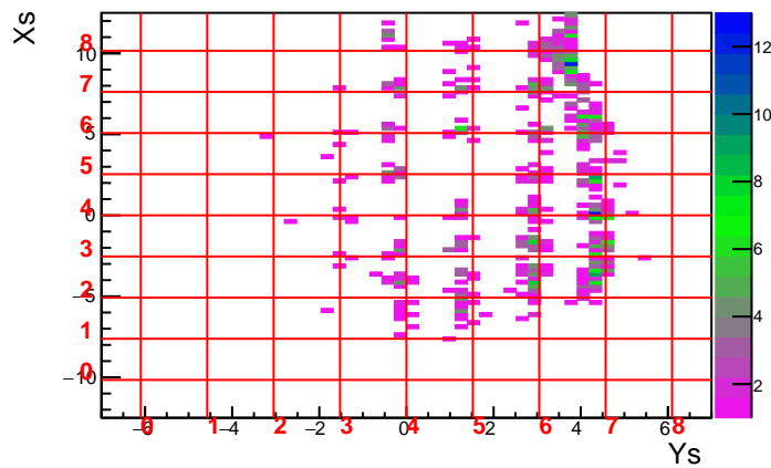
Run 3610 Foil 13.3 DelCut -9.0
