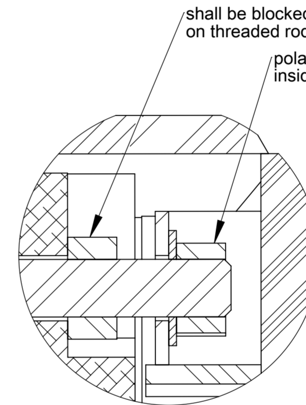
DÉTAIL R ECHELLE 1 : 2
