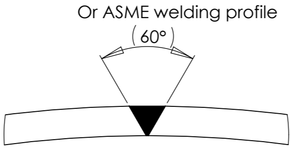
DÉTAIL A ECHELLE 1 : 1
