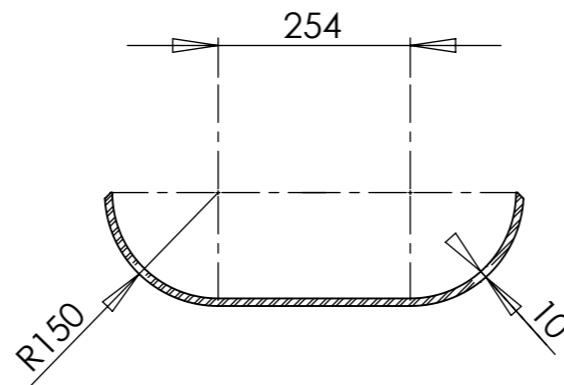
COUPE A-A ECHELLE 1 : 10
