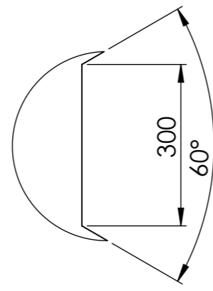
DÉTAIL B ECHELLE 1 : 10
