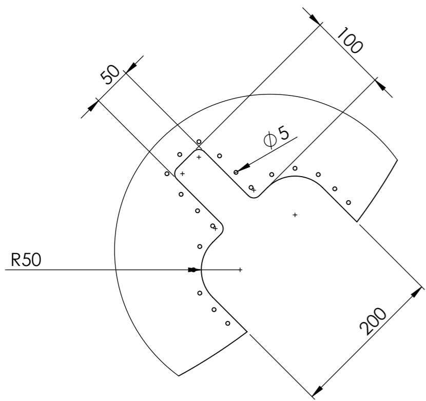
DÉTAIL A ECHELLE 1 : 5
