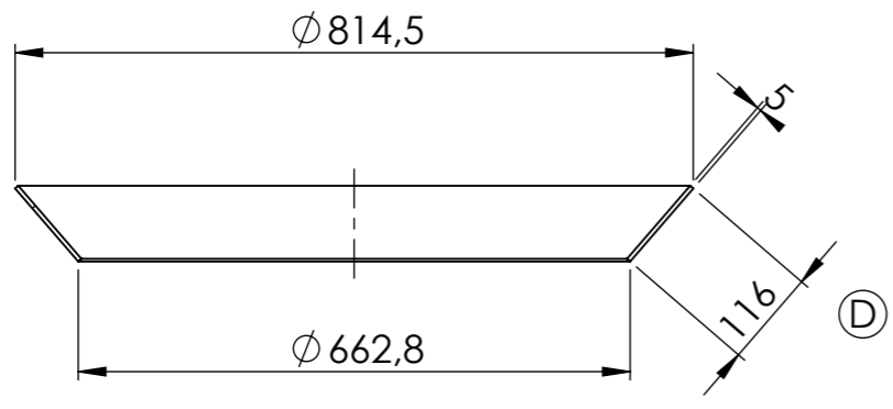
COUPE A-A
