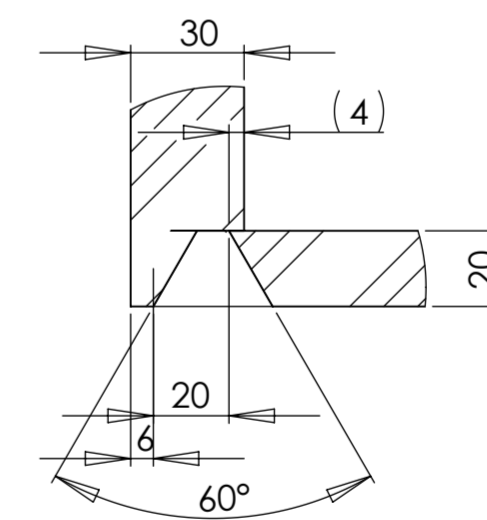
DÉTAIL C ECHELLE 1 : 2
