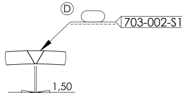
DÉTAIL D ECHELLE 1 : 2
