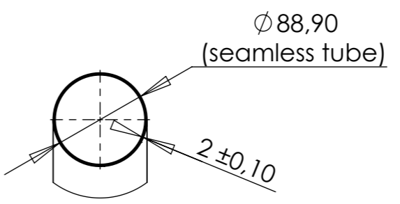
DÉTAIL A ECHELLE 1 : 5
