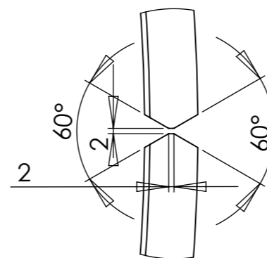
DÉTAIL C ECHELLE 1 : 2
