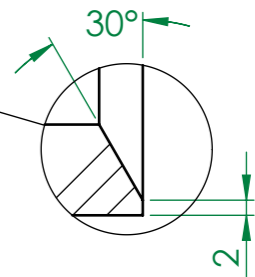
DÉTAIL C ECHELLE 1 : 1
