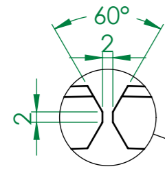
DÉTAIL A ECHELLE 1 : 1
