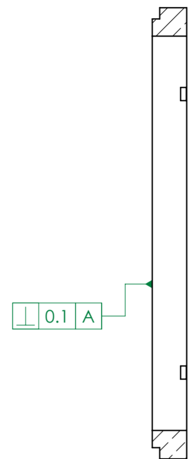
COUPE B-B
