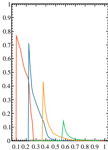
R(e^+e^-)
