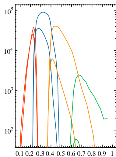
N_{pair} and N_{dis}
