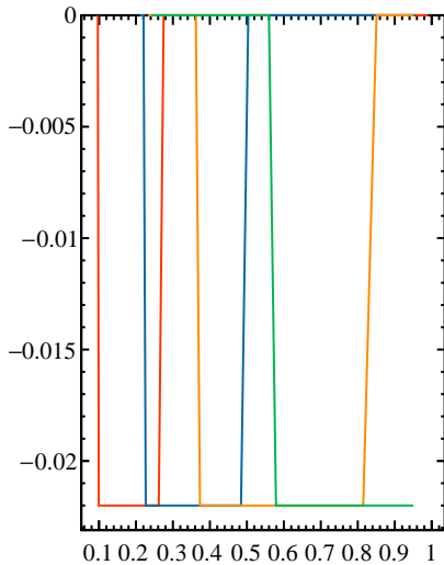
A_{bg}
