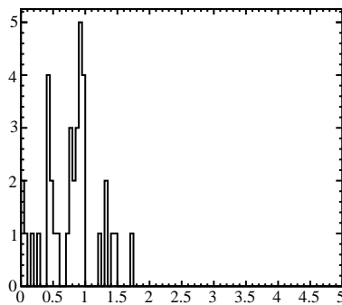
bigalClusters.fCherenkovBestADCSum (TMath::Abs(bigalClusters.fCherenkovTDC)<25)
