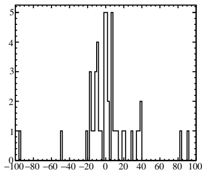
bigalClusters.fCherenkovTDC
