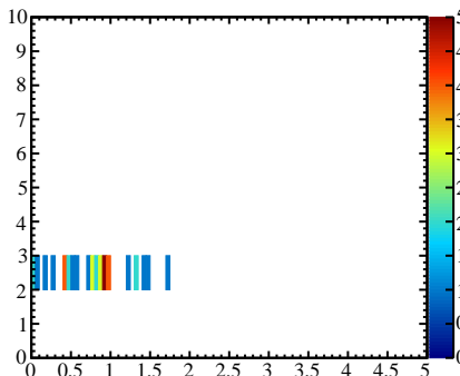
bigalClusters.PrimaryMimicSignalClusters.fCherenkovBestADCSum (TMath::Abs(bigalClusters.fCherenkovTDC)<25)
