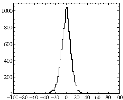
bigalClusters.fCherenkovTDC
