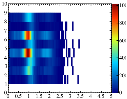
bigalClusters.PrimaryMimicSignalClusters.fCherenkovBestADCSum (TMath::Abs(bigalClusters.fCherenkovTDC)>25)
