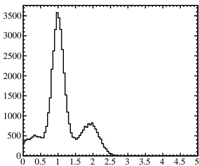
bigalClusters.fCherenkovBestADCSum (TMath::Abs(bigalClusters.fCherenkovTDC)>25)
