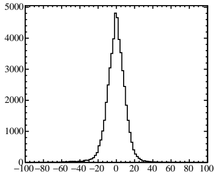
bigalClusters.fCherenkovTDC
