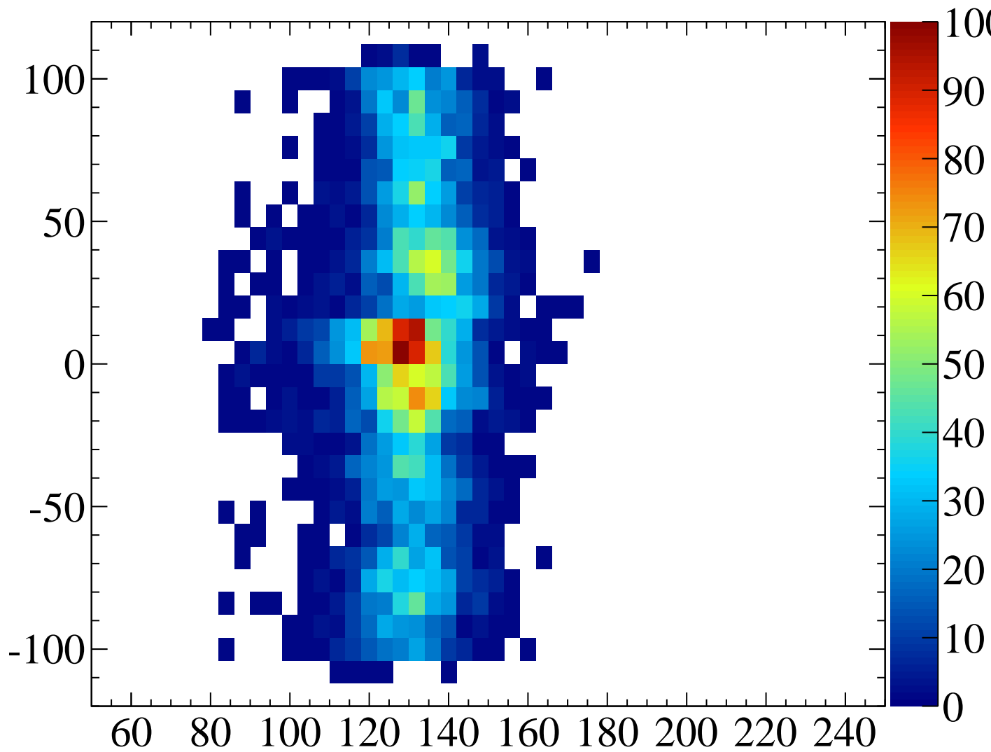
massVSy2
