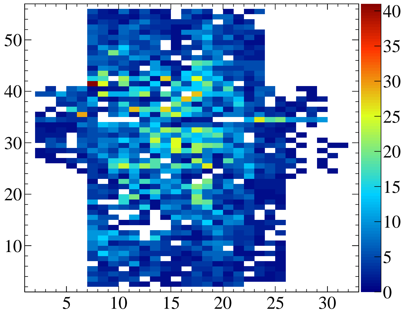
clustxVSy1
