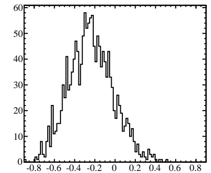
\Delta E
