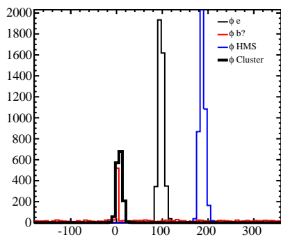
Phi e
