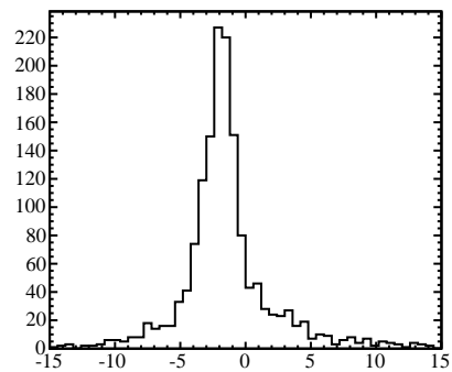
\Delta \phi_e
