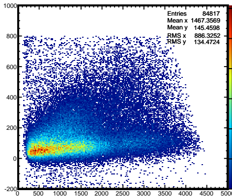
fDelta_Energy:fClusterEnergy
