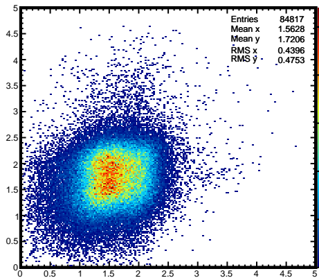
fYClusterSigma:fXClusterSigma
