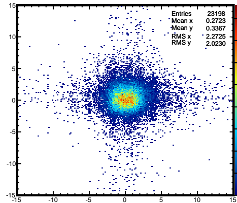
fYClusterSkew:fXClusterSkew
