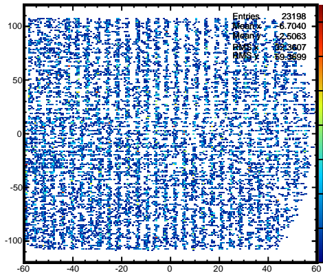
fYCluster:fXCluster
