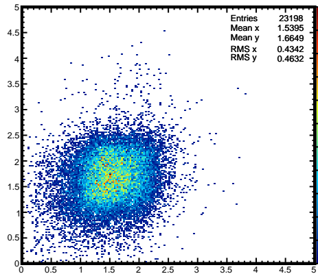
fYClusterSigma:fXClusterSigma
