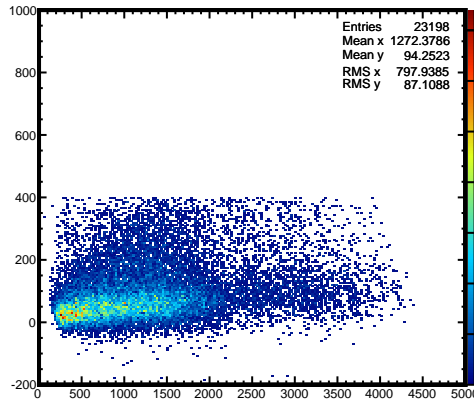
fDelta_Energy:fClusterEnergy
