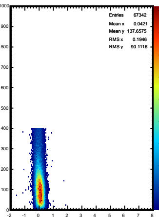
fDelta_Energy:fDelta_Theta*180.0/TMath::Pi()
