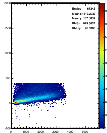
fDelta_Energy:fClusterEnergy
