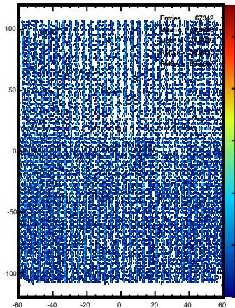
fYCluster:fXCluster
