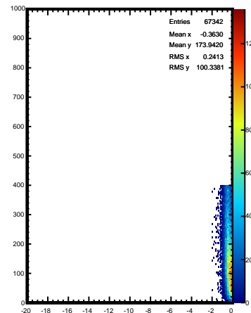
fDelta_Energy:fDelta_Phi*180.0/TMath::Pi()
