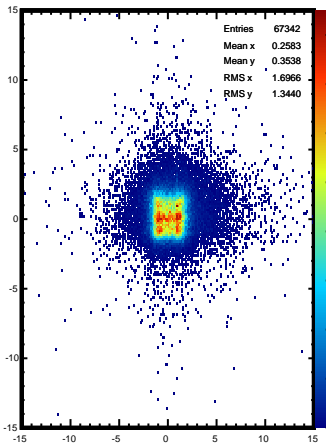
fYClusterSkew:fXClusterSkew
