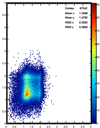
fYClusterSigma:fXClusterSigma
