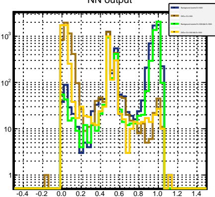
NN output
