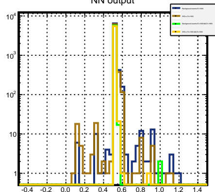
NN output
