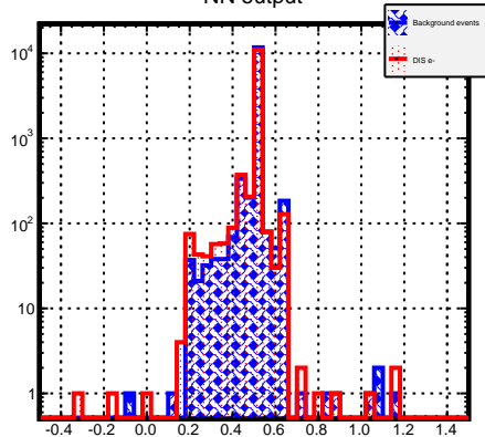
NN output
