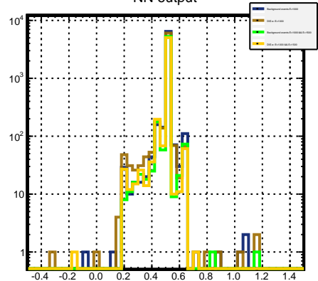
NN output
