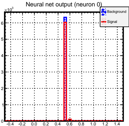
NN output
