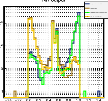
NN output
