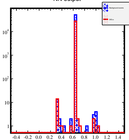
NN output
