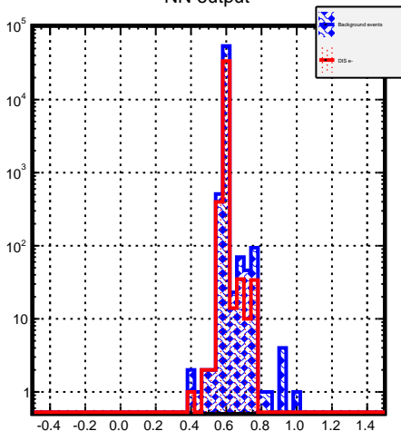
NN output
