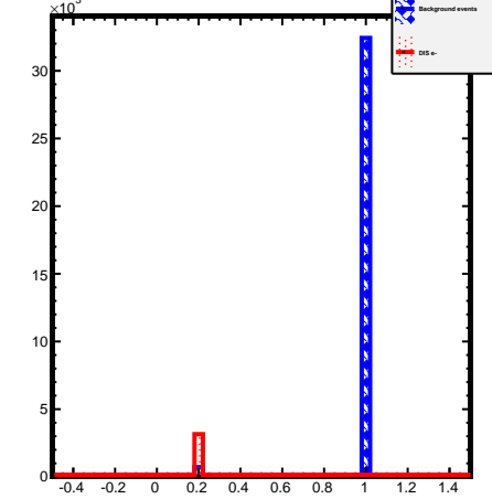
NN output
