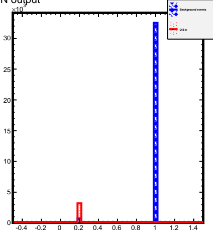
NN output
