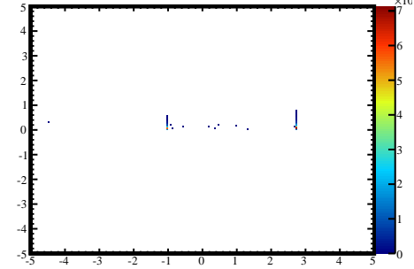
\Delta y test
