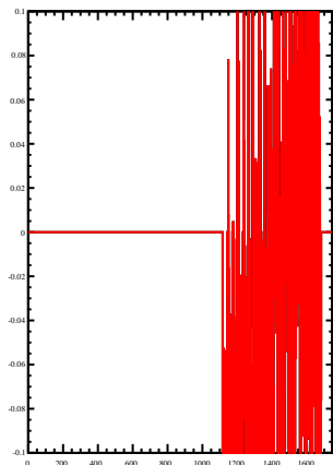
fEpsilonHist
