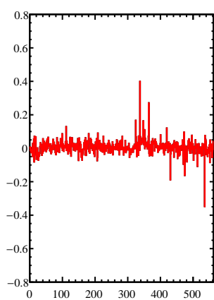
fEpsilonHist
