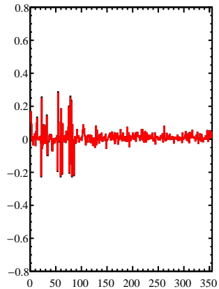
fEpsilonHist
