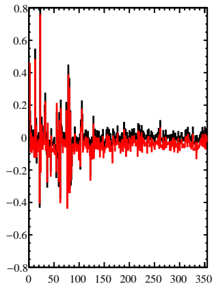
fEpsilonHist
