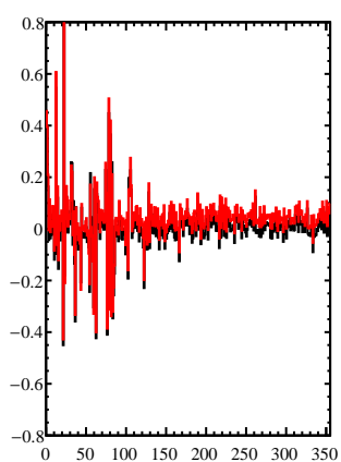
fEpsilonHist
