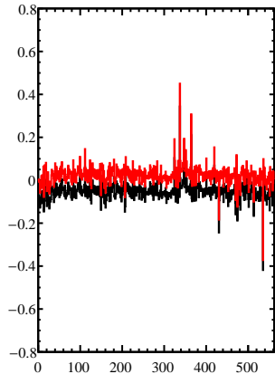
fEpsilonHist
