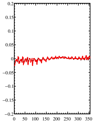
fEpsilonHist
