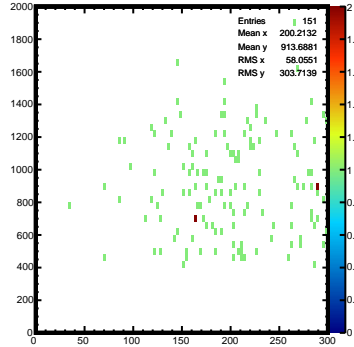
E1 vs \pi mass
