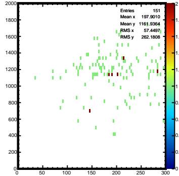
E2 vs \pi mass
