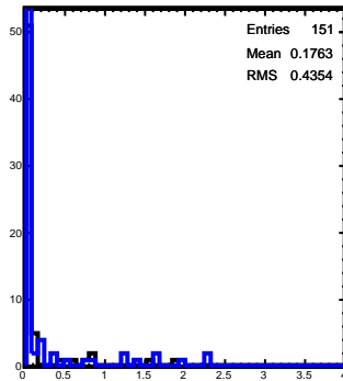
Positron Cer
