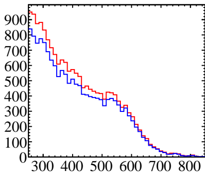
mass3
