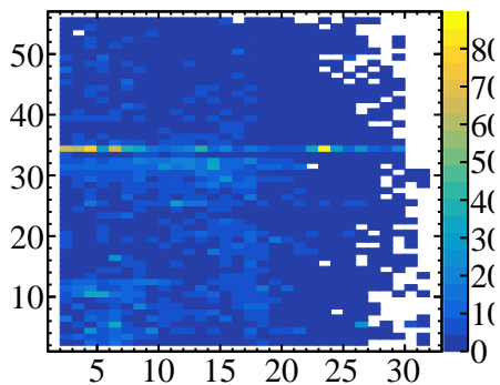
clustxVSy1
