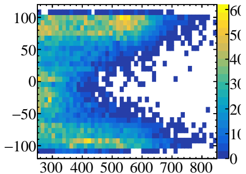
massVSy2
