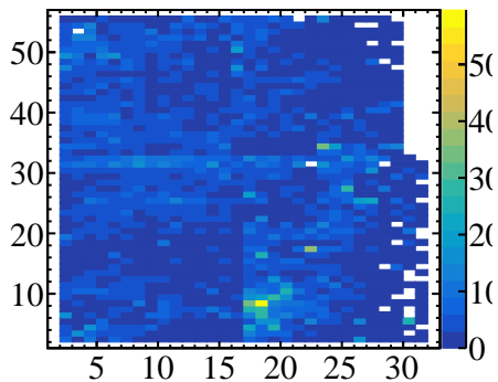
clustxVSy2
