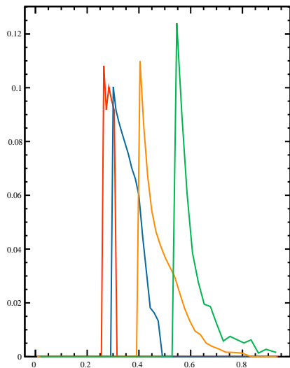
R(e^+e^-)
