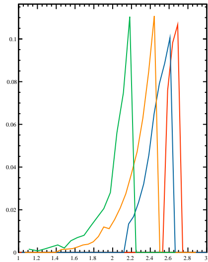
R(e^+/e^-)
