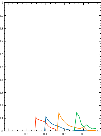
R(e^+/e^-)
