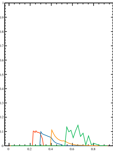
R(e^+e^-)
