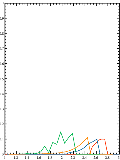
R(e^+e^-)
