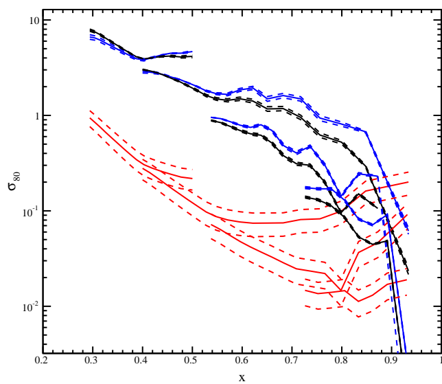
\sigma_{80}, E=4.7 \text{ GeV}
