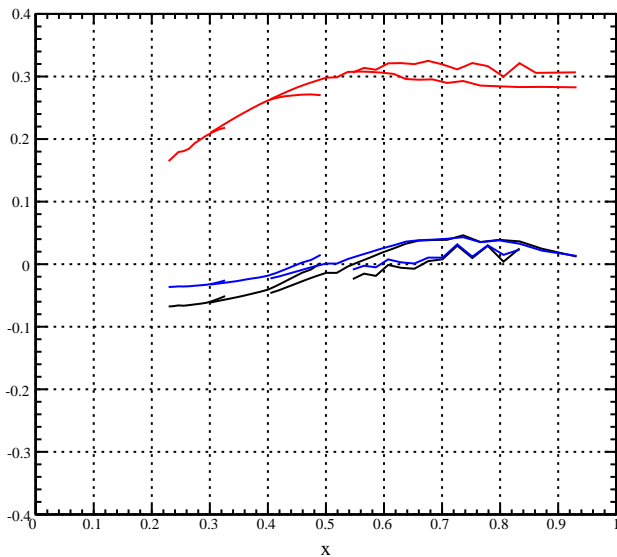
A_{80}, E=5.9 \text{ GeV}
