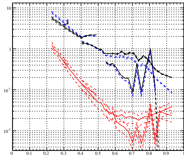
\sigma_{80}, E=5.9 \text{ GeV}
