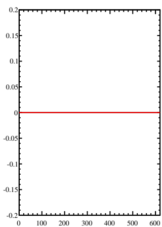
fEpsilonHist
